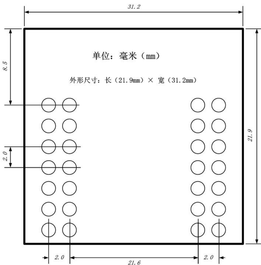
图 4: GC-02-DIP 机械尺寸图
