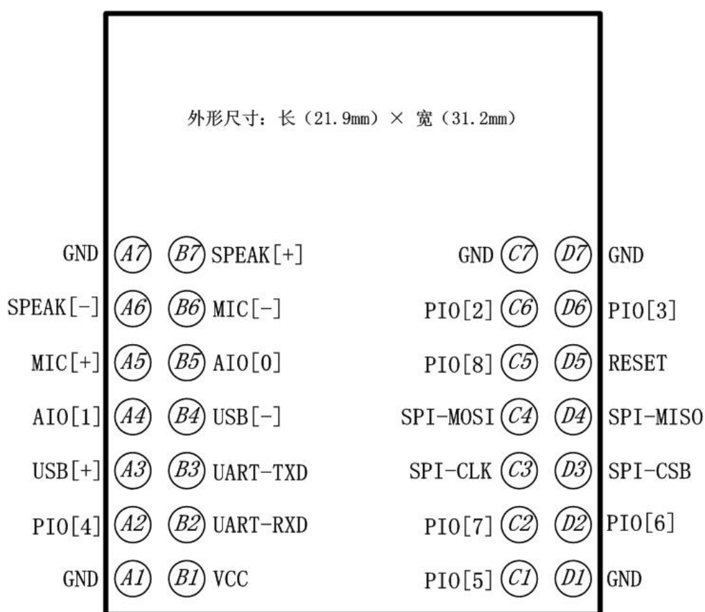
图 5: GC-02-DIP 引脚定义图
