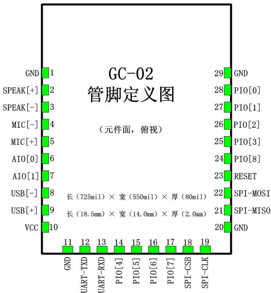
图 3: GC-02 引脚定义图
