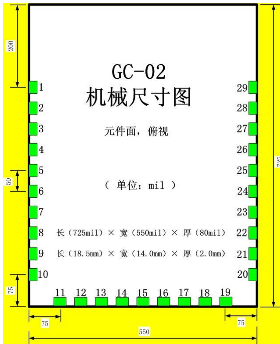
图 2: GC-02 模块机械尺寸图
